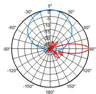
690-960MHz(65 deg)
